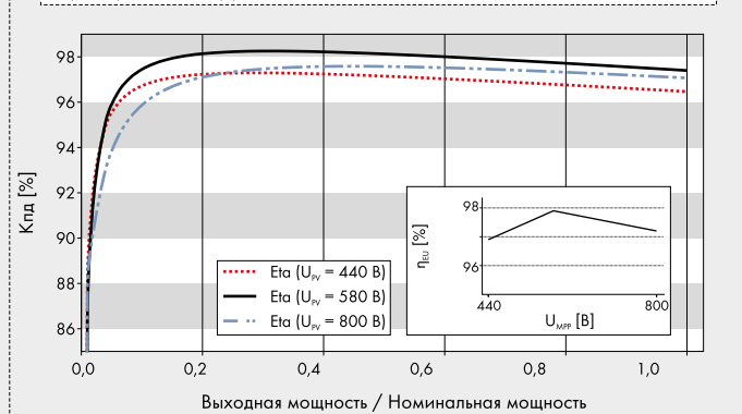
Характеристика коэффициента полезного действия SUNNY TRIPOWER 12000TL
